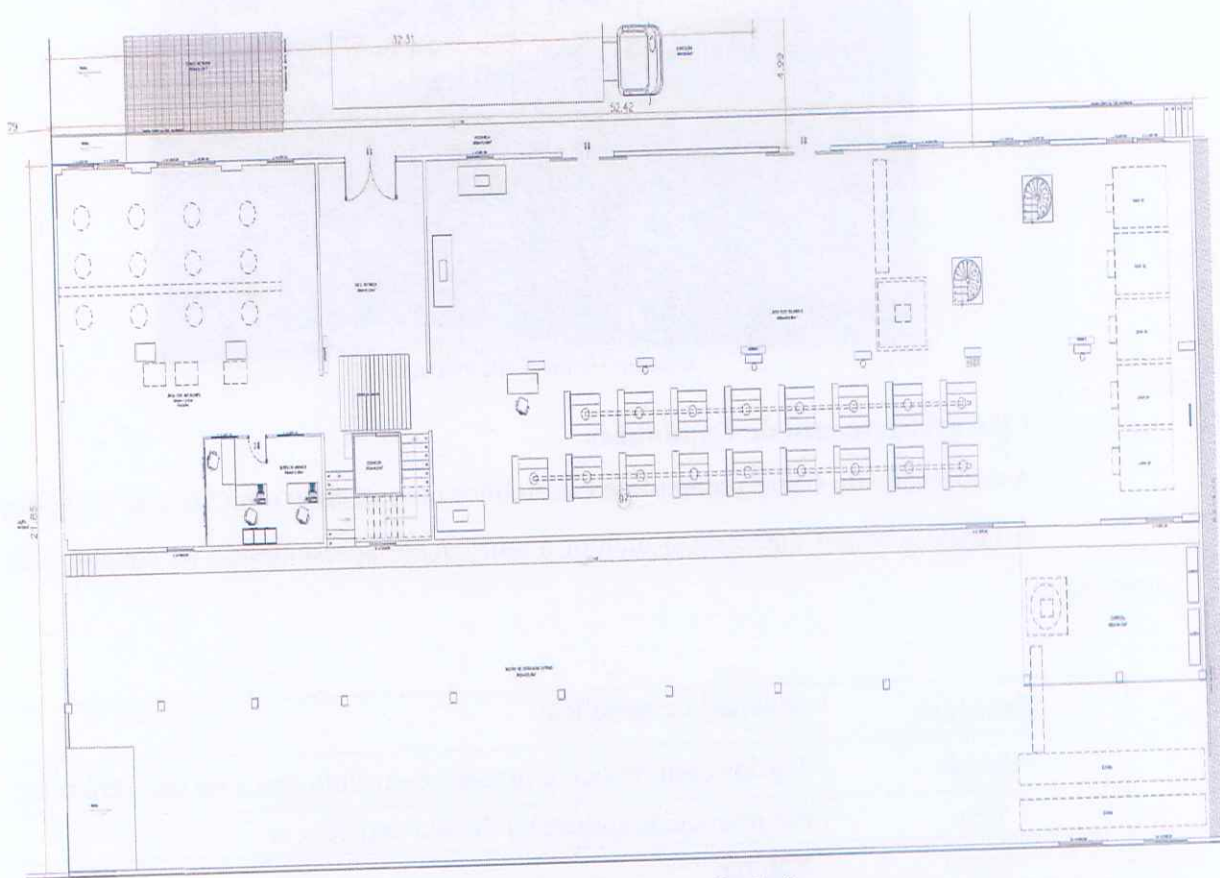
Imagem 18: Planta Baixa – Produção
